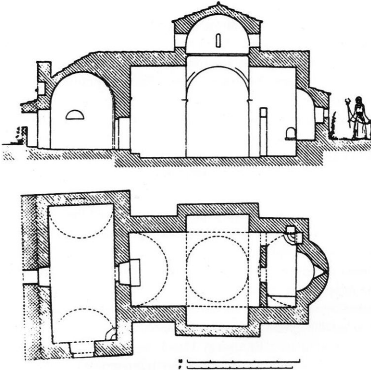
Τομή κατά μήκος και κάτοψη του ναού της Κοιμήσεως της Θεοτόκου στο Παλιοχώρι. (Από το βιβλίο Χ. Μπούρα - Αθ. Καλογεροπούλου, Εκκλησίες της Αττικής, Αθήνα 1969, σχέδιο XXIX).
