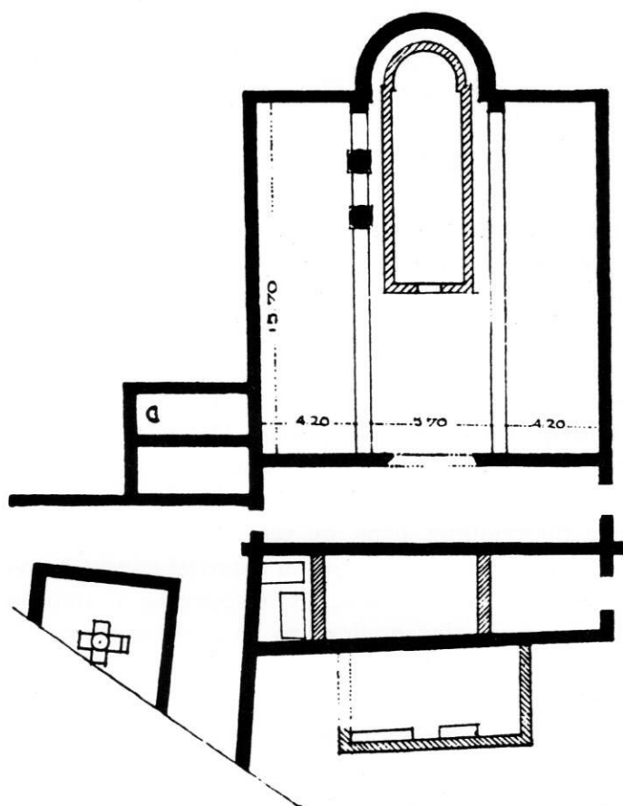
Κάτοψη παλαιοχριστιανικής βασιλικής της Ελευσίνας στη θέση όπου σήμερα ο μεταβυζαντινός ναΐσκος του Αγίου Ζαχαρία (Αναδημοσιεύεται από τη μελέτη του Γ. Σωτηρίου, Αί παλαιοχριστιανικά βασιλικά της Ελλάδος, «'Αρχαιολογική 'Εφημερίς» 1929, σ. 184).
