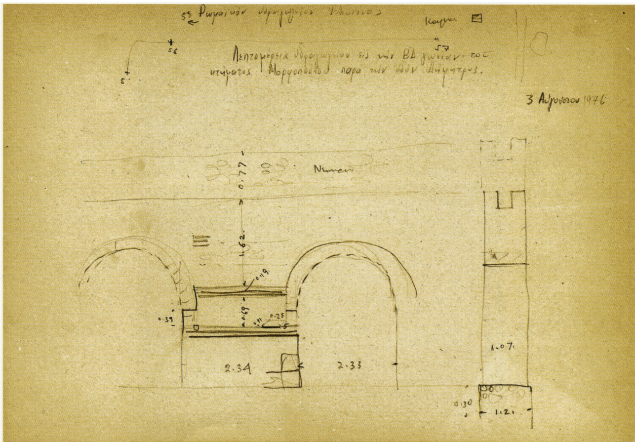
Σκίτσο αποτύπωσης του υδραγωγείου (Ι. Τραυλός 1976, ΑΑΕ Αρχείο Ι. Τραυλού)
