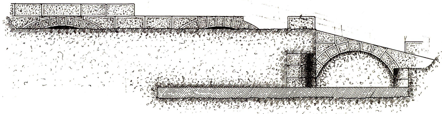
Σχέδιο αποτύπωσης της βόρειας όψης της γέφυρας, πριν από την ανασκαφή (Ι. Τραυλός, ΑΑΕ, Αρχείο Ι. Τραυλού, αρ. ΙΙ39)
