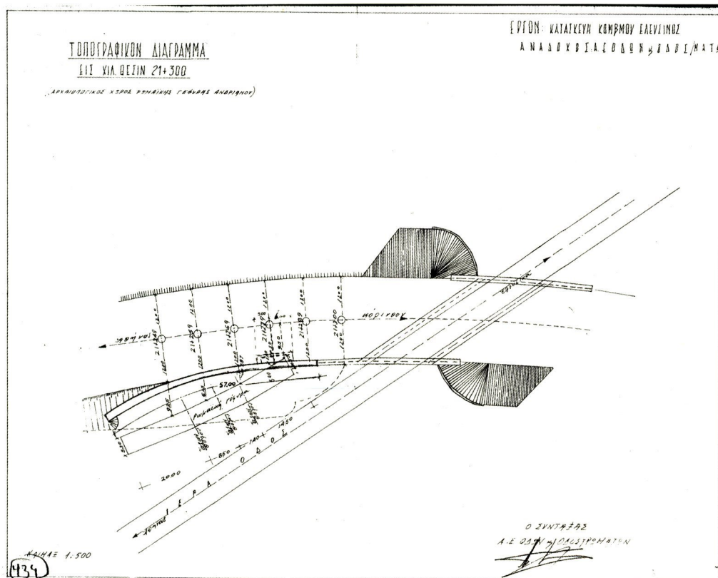
Τοπογραφικό διάγραμμα του ανισόπεδου κόμβου της Εθνικής Οδού πάνω από την αρχαία γέφυρα (ΑΑΕ, Αρχείο Ι. Τραυλού, αρ. ΙΙ56)
